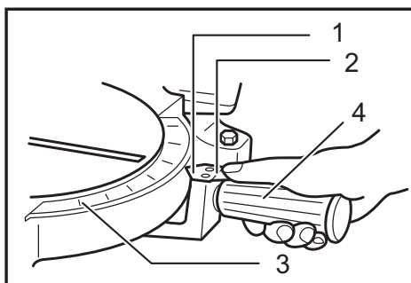
► 1. Pointer 2. Lock lever 3. Miter scale 4. Grip
