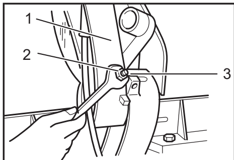
► 1. Carter d'engrenage 2. Écrou hexagonal 3. Boulon de réglage
