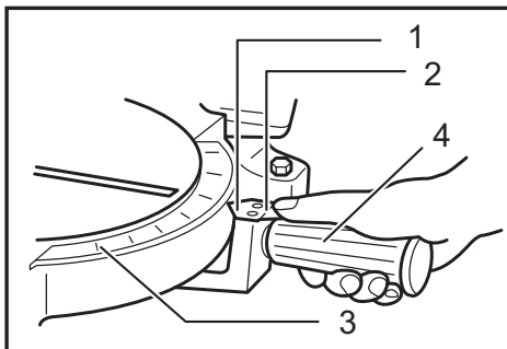
► 1. Index 2. Levier de verrouillage 3. Échelle de coupe d'onglet 4. Poignée
