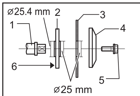
► 1. Spindle 2. Inner flange 3. Blade 4. Outer flange 5. Hex bolt 6. 25.4 mm marking
