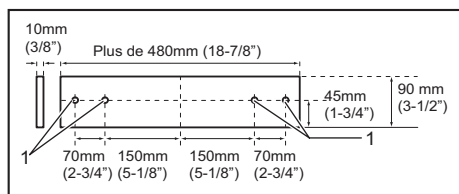
► 1. Orifice
